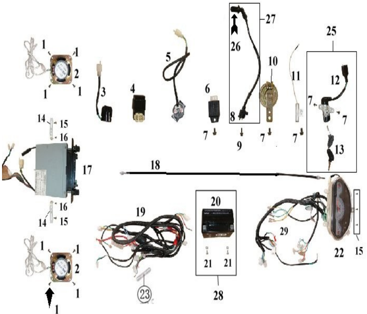
Touring 150 DE Diagram 2 ---- Cables & wiring
